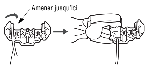
Fil de connexion de frein à main (frein de stationnement) (Vert clair)
