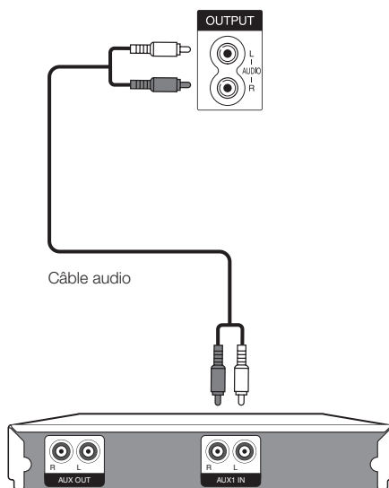
Amplificateur avec entrée audio analogique
