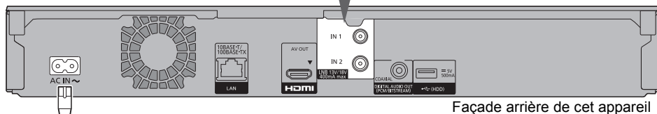
Façade arrière de cet appareil
