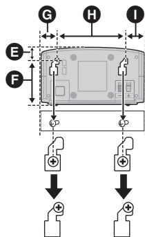
Enceinte centrale
