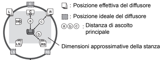
Cerchio della distanza di ascolto primaria costante
