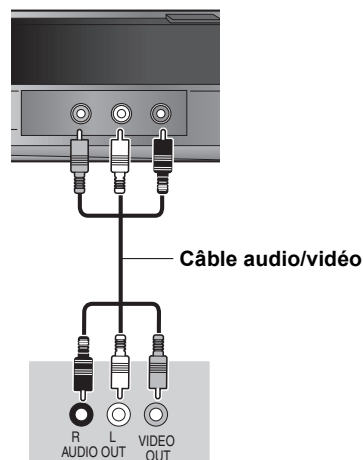
Face arrière du magnétoscope
