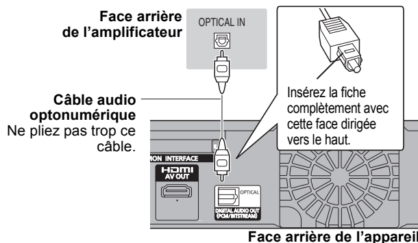
Face arrière de l'appareil
