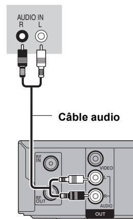
Face arrière de l'appareil
