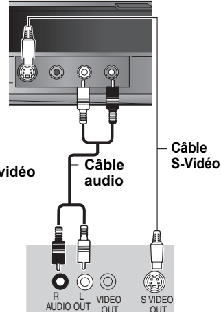
Face arrière du magnétoscope
