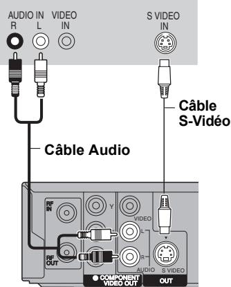
Face arrière de l'appareil
