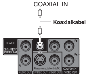
Rückseite des DVD-Spielers
