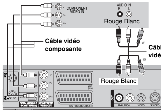
Face arrière de l'appareil
