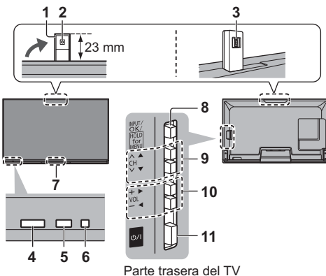
Parte trasera del TV
