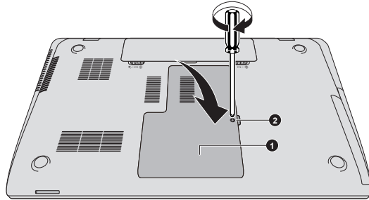
Illustration 4-10 Retrait du capot du module mémoire
