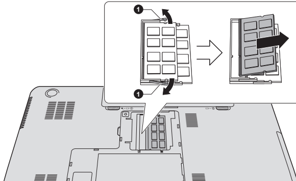
Illustration 3-15 Retrait d'un module mémoire
