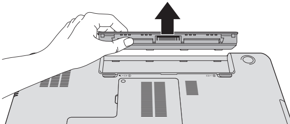
Illustration 5-2 Retrait de la batterie - 2
