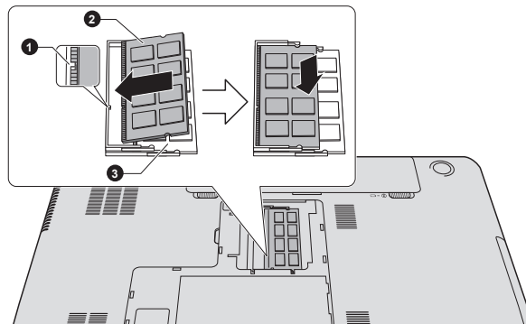
Illustration 3-13 Pose du module mémoire
