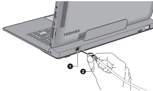
Illustration 4-16 Branchement du câble réseau
