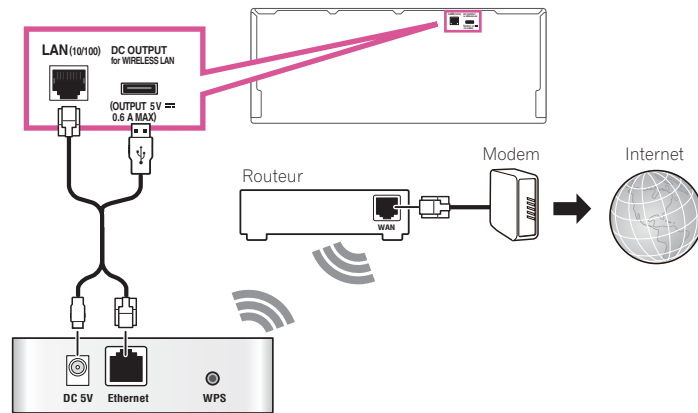
Convertisseur LAN sans fil (AS-WL300)
