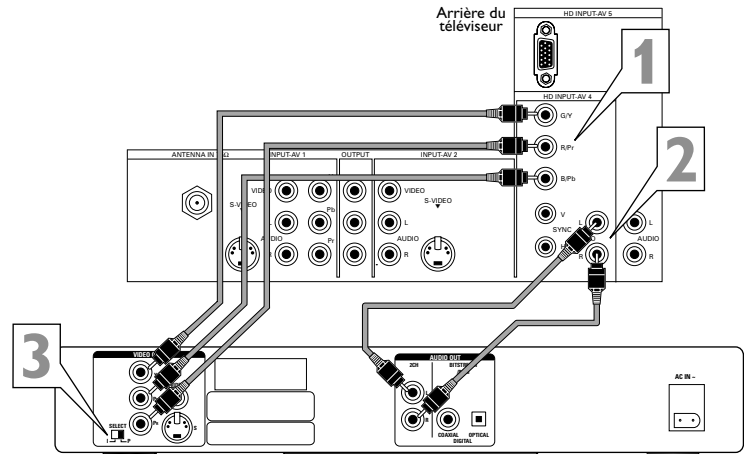
Arrière du lecteur DVD à balayage progressif
