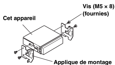
Applique de montage
