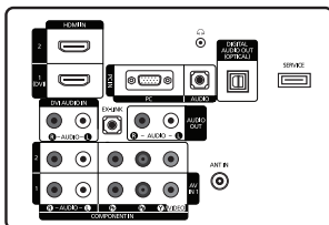
DÉTAILS DU PANNEAU DE PRISES 5.2"H X 6.6"W
