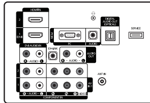
DÉTAILS DU PANNEAU DE PRISES 5.2" H X 6.6" W
