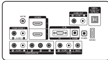
DÉTAILS DU PANNEAU DE PRISES 5.2" H X 6.6" W
