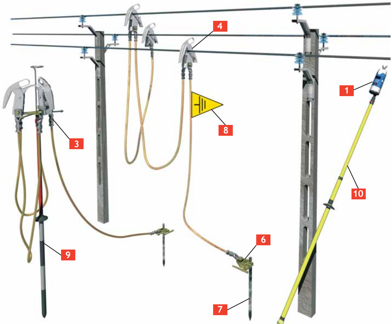
Système de mise à la terre et en court-circuit
