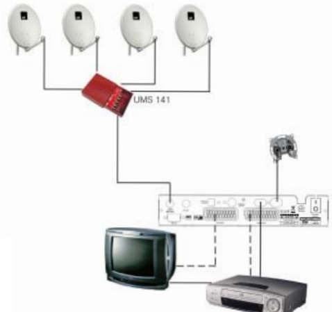
Exemple 2 - Commutateur DISEqC
