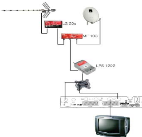
Exemple 3 - Mélange avec le terrestre
