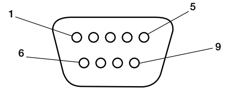
Mini D-SUB 9 clavijas
