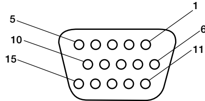
Mini D-sub 15 clavijas
