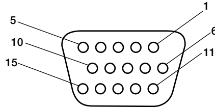
Mini D-SUB à 15 broches
