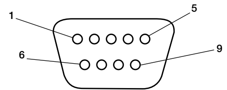
Mini D-SUB 9P
