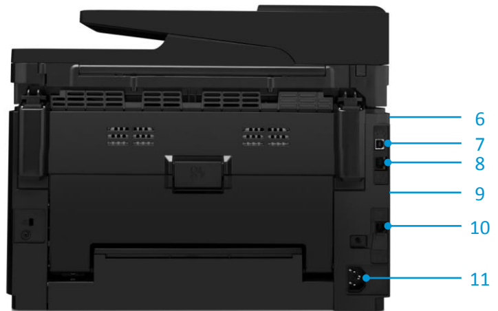
Vue arrière
