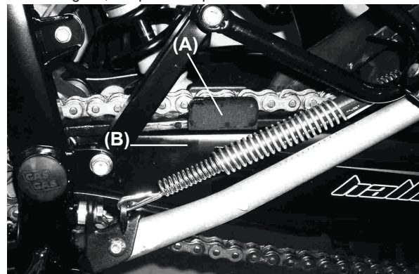
(A). Patin de guide de chaîne. (B). Bras basculeur.
