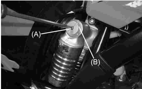
(A). Ajusteur de haute compression. (B). Ajusteur de basse compression.
