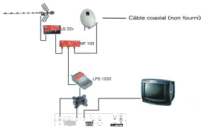
Exemple 3 – Mélange avec le terrestre
