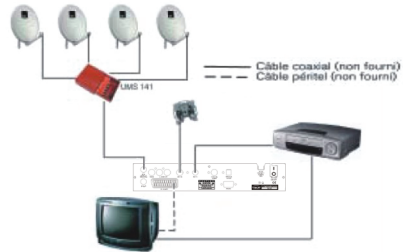
Exemple 2 – Commutateur DISEqC
