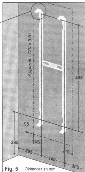
Fig. 5 Distances en mm
