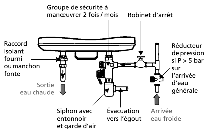
Schéma de raccordement (exemple d'un vertical mural)
