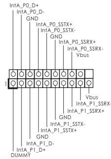
USB 3.0 扩展接头 (19 针 USB3_3_4) (见第 2 页第 8 项)
