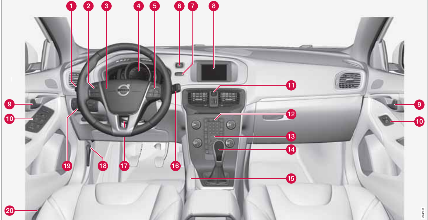
Conduite à gauche.
