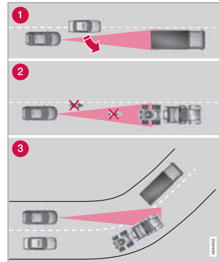
Champ de vision de l'ACC.
