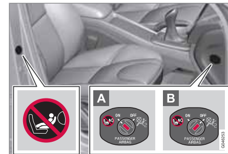
Emplacement de l'autocollant et du commutateur de coussin gonflable.
