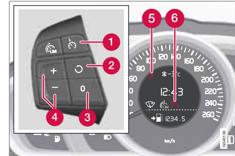
Clavier au volant et écran dans une voiture avec limiteur de vitesse 1 .
