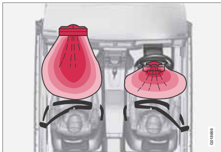
Systeme de coussin gonflable vu du dessus, voiture avec conduite à droite.
