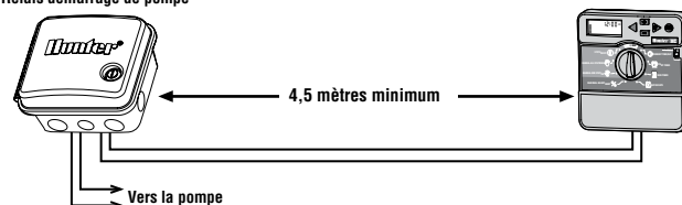
Séries PSR Relais démarrage de pompe
