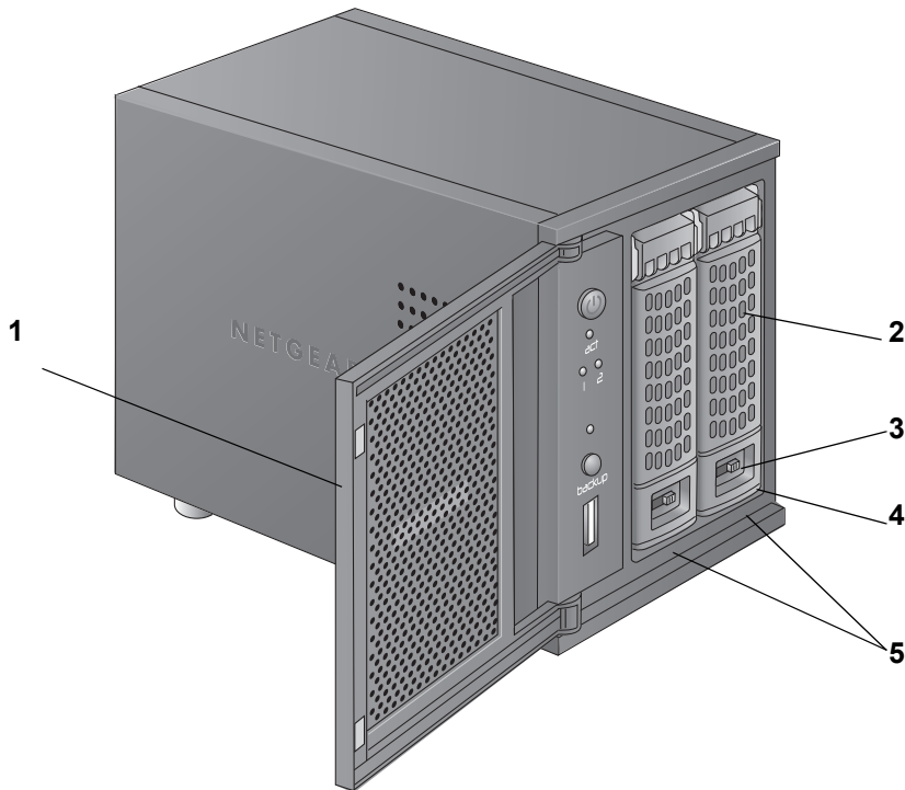
Figure 2. Baies de lecteur du ReadyNAS Duo v2
