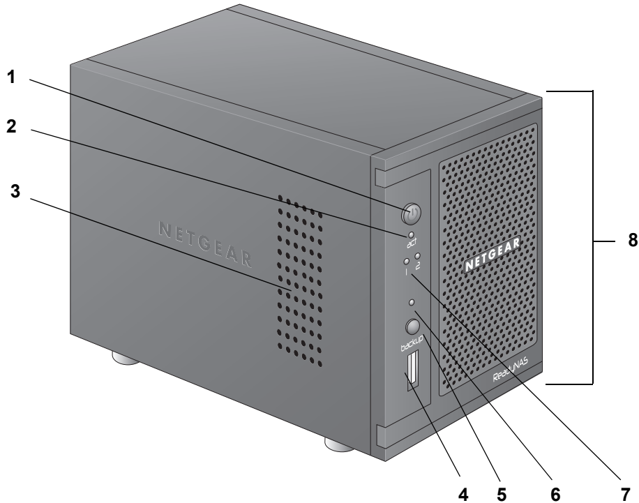
Figure 1. Panneaux avant et latéral du ReadyNAS Duo v2
