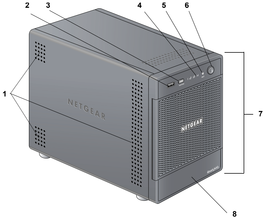
Figure 5. Panneaux avant et latéral du ReadyNAS NV+ v2
