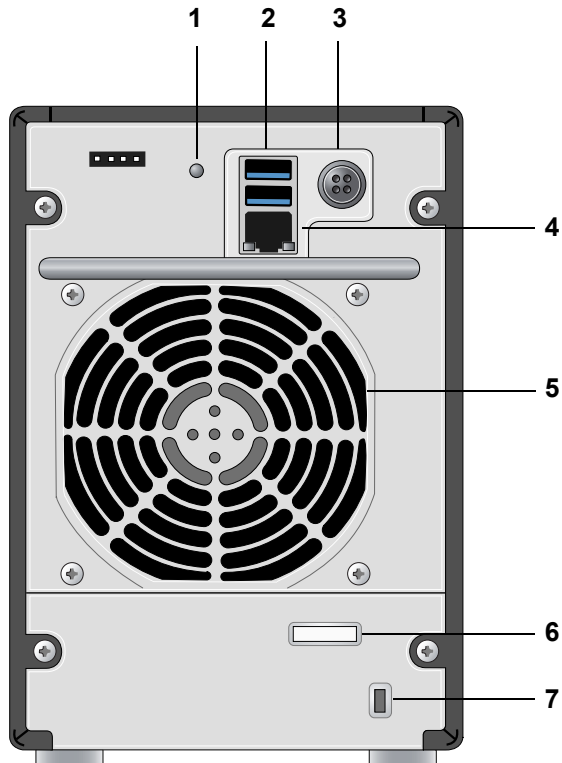
Figure 8. Panneau arrière du ReadyNAS NV+ v2
