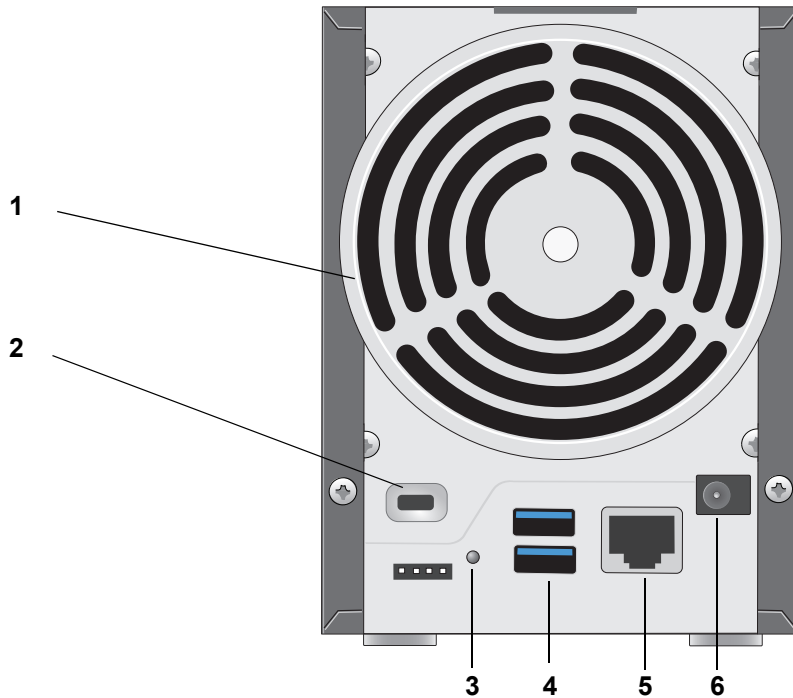
Figure 4. Panneau arrière du ReadyNAS Duo v2
