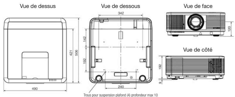
Trous pour suspension plafond (4) profondeur max 10
