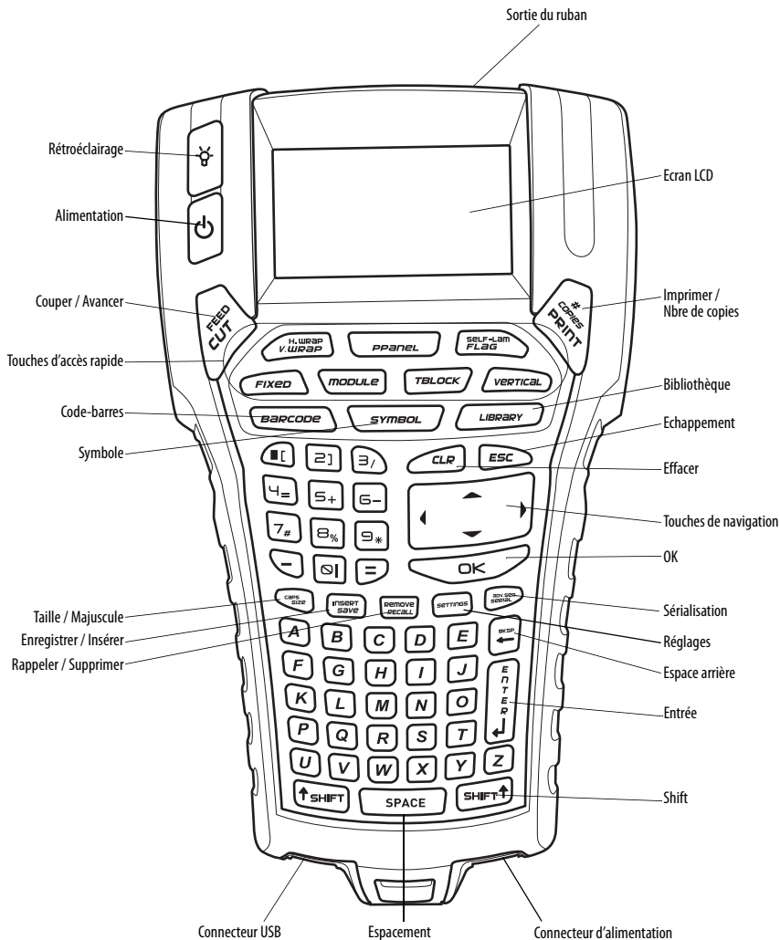
Figure 1 Imprimante RHINO 6000
