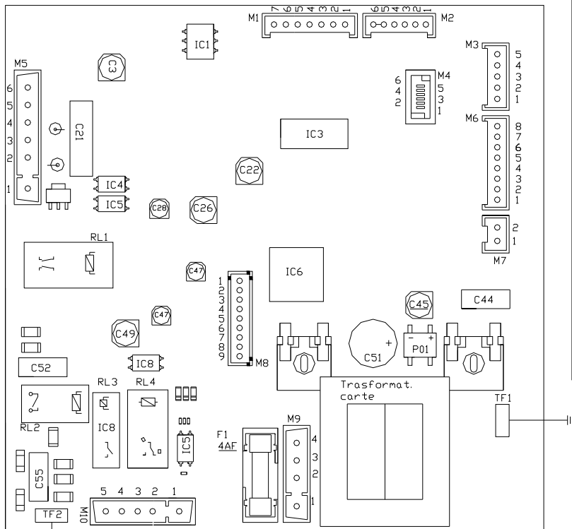
CARTE ELECTRONIQUE DIGITECH - SM 20019 COD. 76677LA
