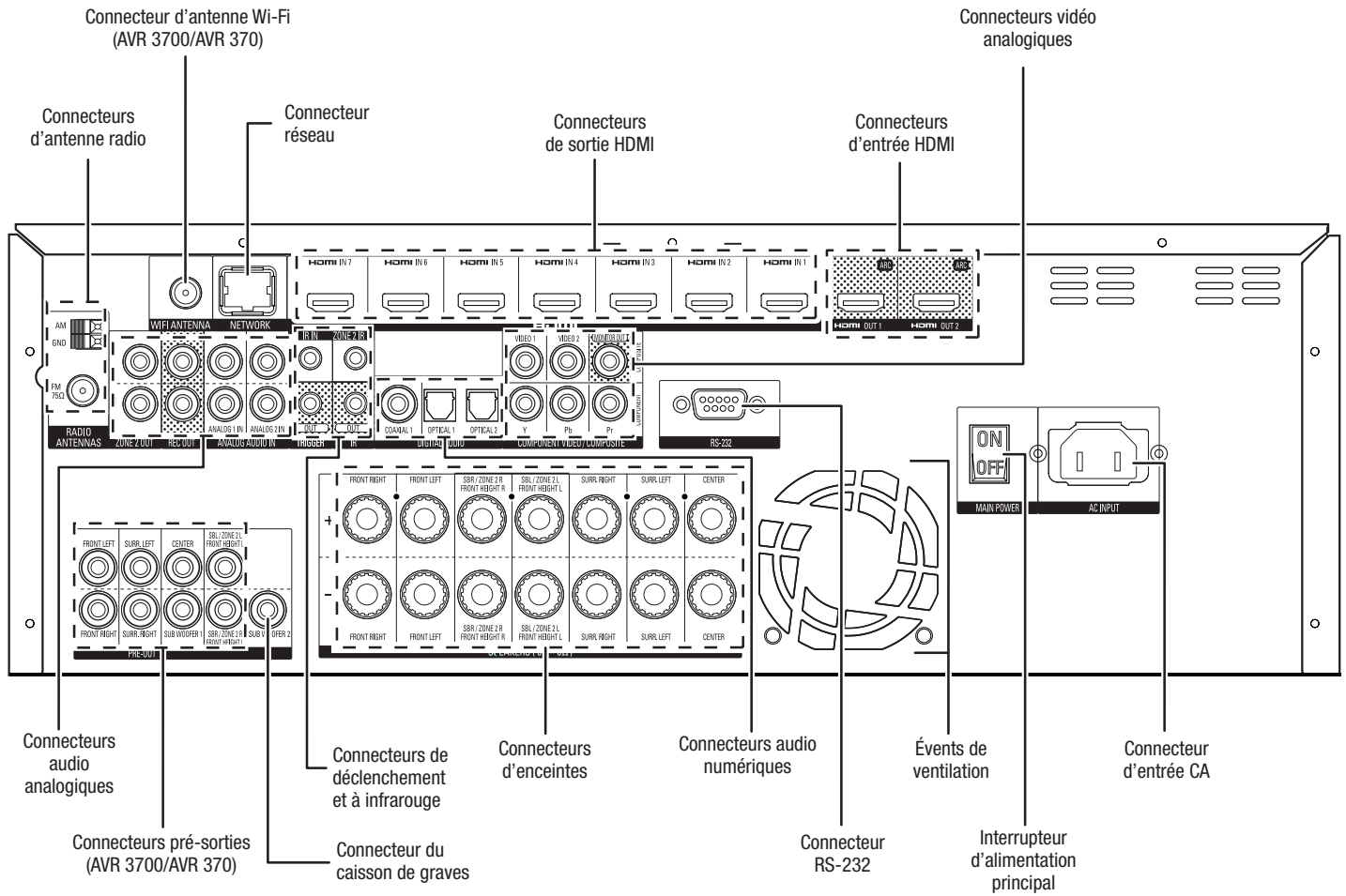
Connecteurs du panneau arrière (illustration AVR 3700)
