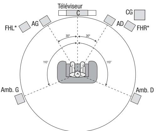
Positionnement des enceintes pour les systèmes à canaux 7.1
