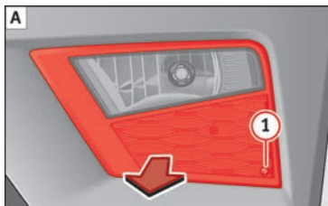
Fig. 107 Phare antibrouillard : dépose du support d'ampoule
