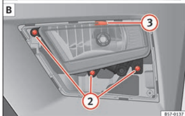
Fig. 106 Phare antibrouillard : enlever la grille.
