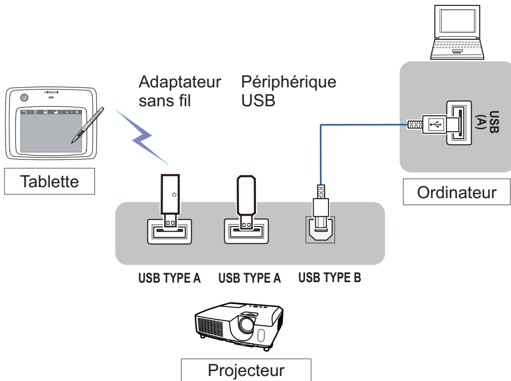
Fig.2 Exemple de connexions
