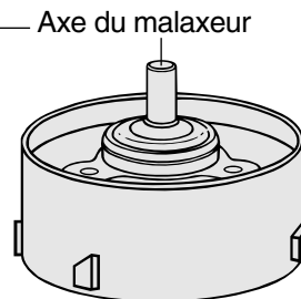
Axe du malaxeur Bloc de fixation de l'axe du malaxeur (N°réf. ADA 29A115)
