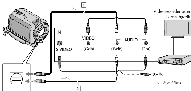
A/V-/Fernbedienungsanschluss
