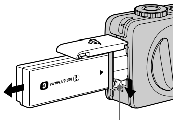
Akkuauswerfhebel
