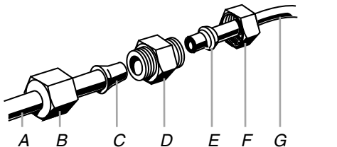
A. Conduit vers le réfrigérateur B. Écrou (fourni) C. Renflement D. Raccord (à acheter) E. Virole (à acheter) F. Écrou (à acheter) G. Canalisation d'eau du domicile
