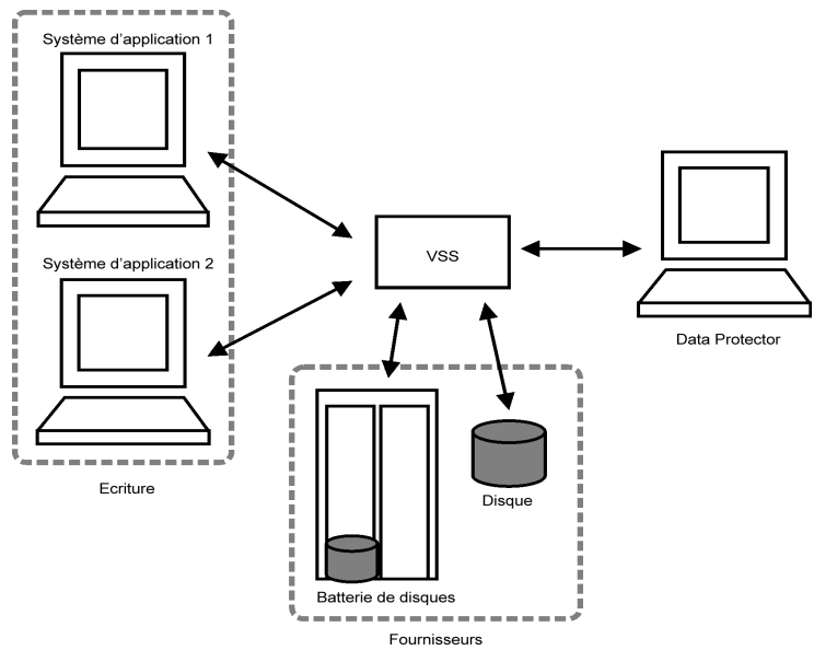
Figure 12-2 Acteurs du modèle de sauvegarde VSS
