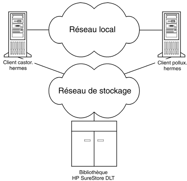
Figure 3-16 Accès direct à la bibliothèque
