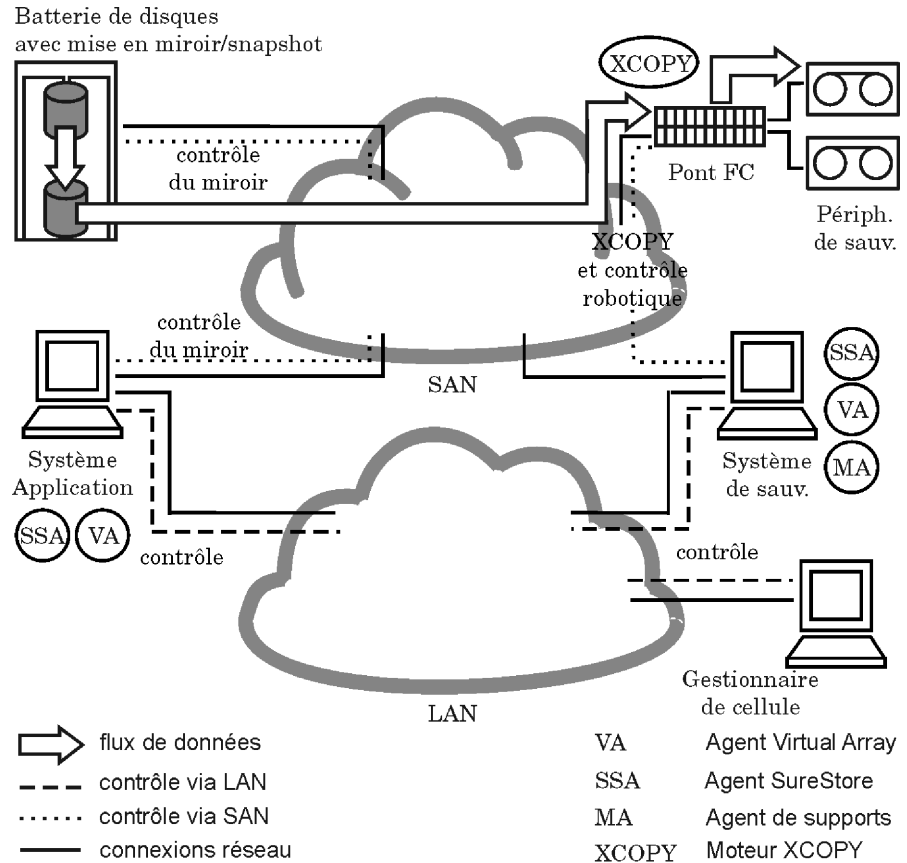
Figure 9-2 Configuration de base à trois hôtes
