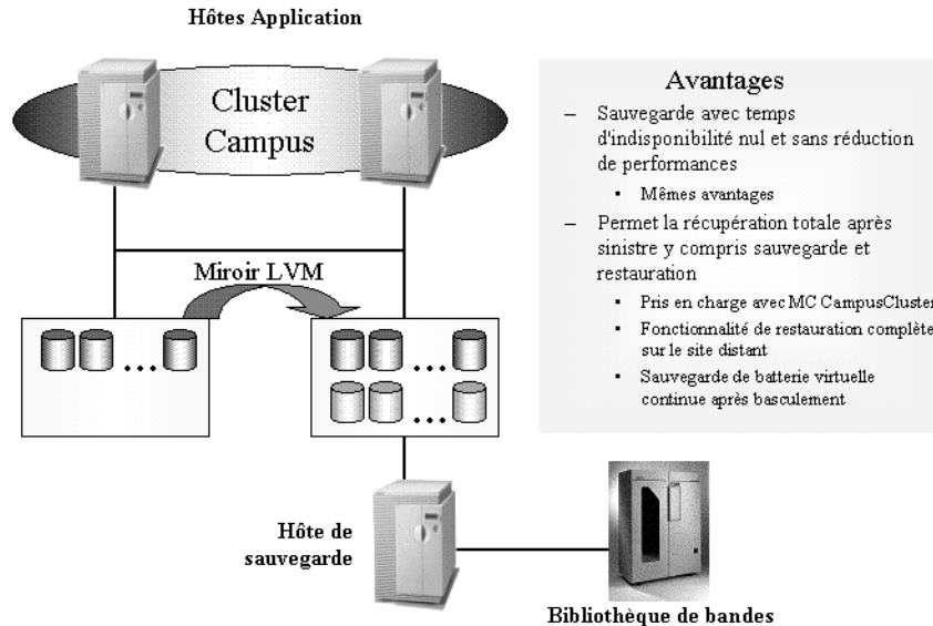
Figure 11-7 Campus Cluster et mise en miroir LVM - HP StorageWorks Virtual Array uniquement
