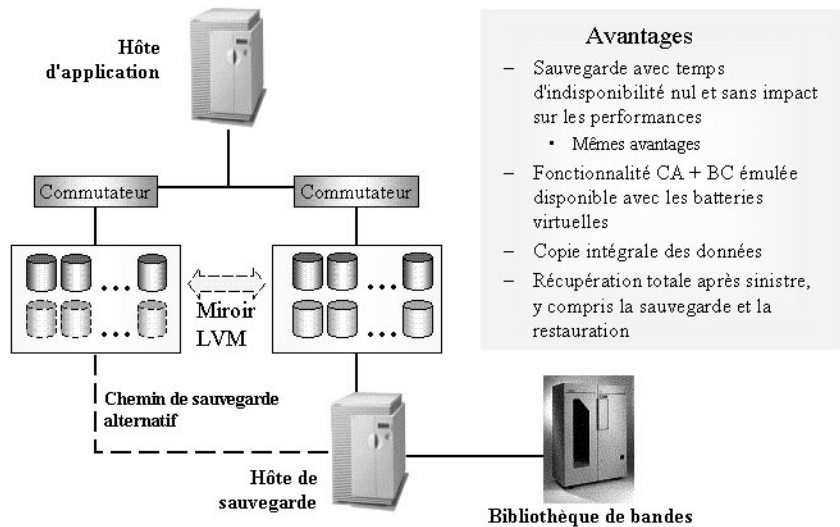
Figure 11-6 Mise en miroir LVM - HP StorageWorks Virtual Array uniquement
