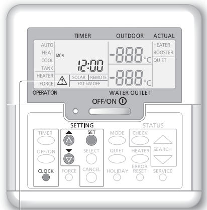
Waarschuwingindicator (tanktemperatuur boven 60 °C)
