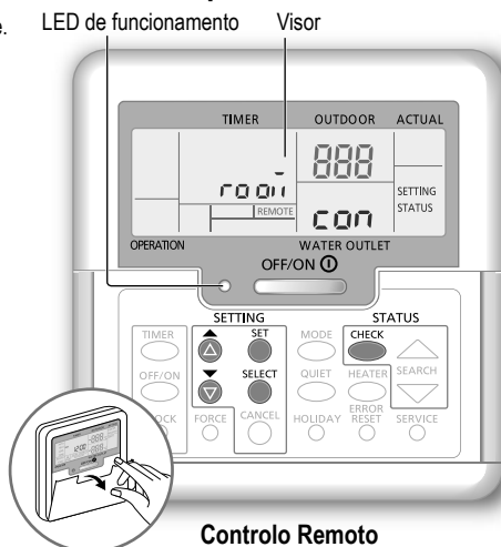
Controlo Remoto
