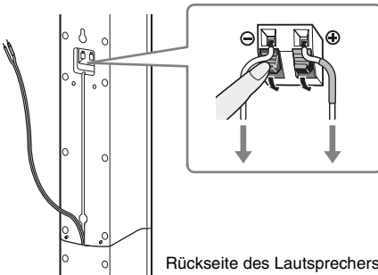
Rückseite des Lautsprechers
