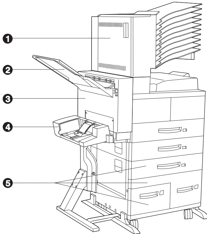
Figure 1.3 Éléments remplaçables par le client
