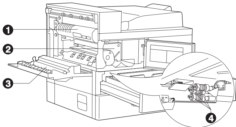
Figure 1.3 Éléments remplaçables par le client
