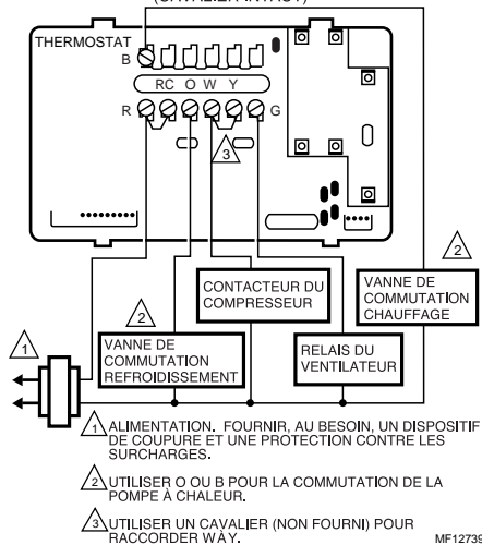
4 FILS – POMPE À CHALEUR À UN ÉTAGE (CAVALIER INTACT)
