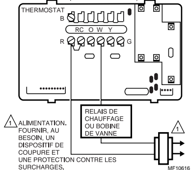
2 FILS – CHAUFFAGE SEULEMENT (CAVALIER INTACT)
