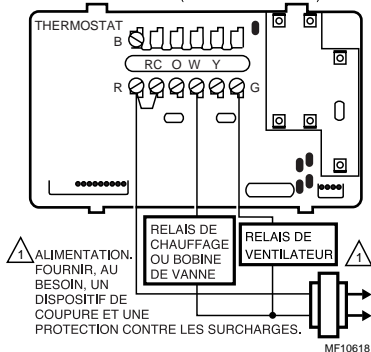
3 FILS - CHAUFFAGE SEULEMENT AVEC VENTILATEUR (CAVALIER INTACT)
