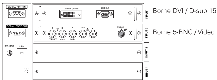
BORNES D'ENTREE/SORTIE
