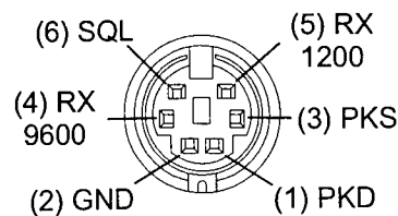
Vue de la façade arrière
