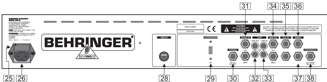
Fig. 1.2: Les connexions sur la face arrière
