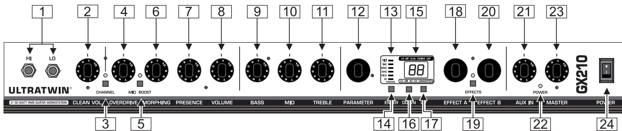
Fig. 1.1: Éléments de contrôle de la façade
